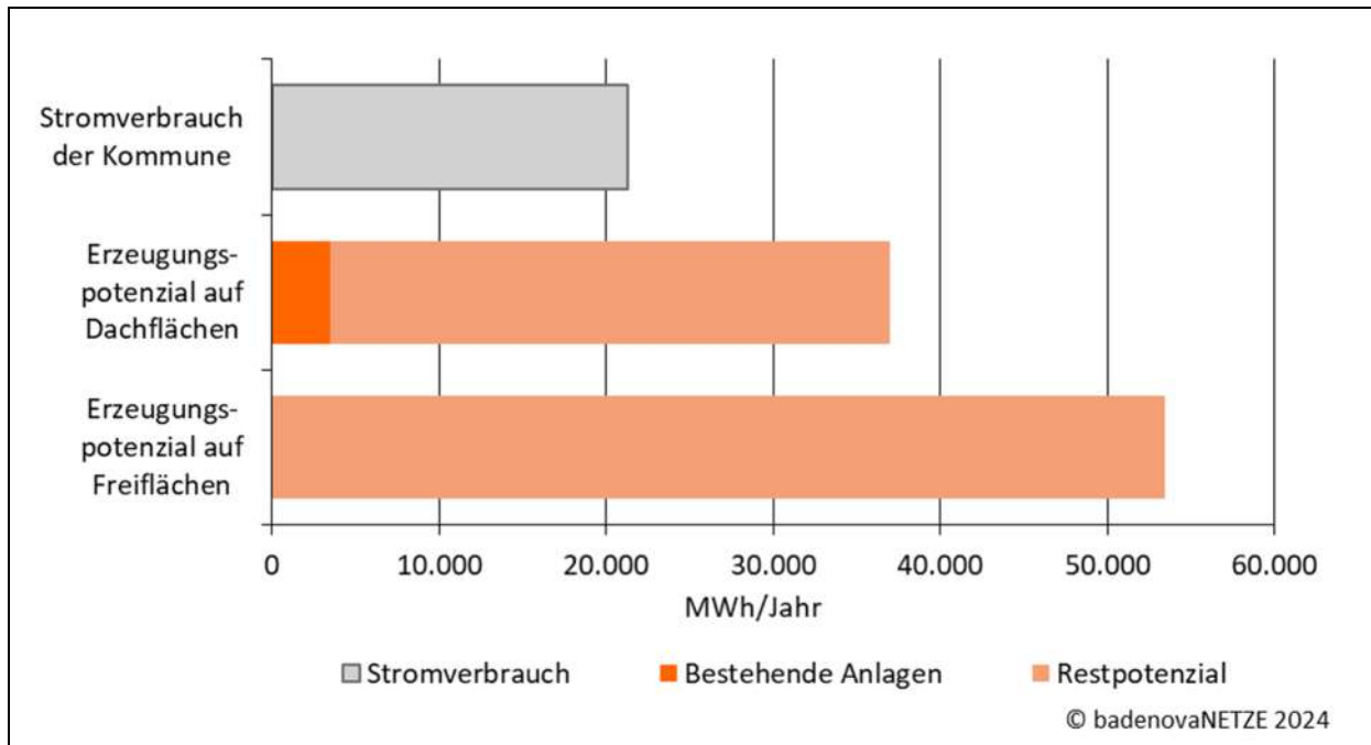
Abbildung 17 – Stromezeugungspotenziale mit PV in Ehrenkirchen
