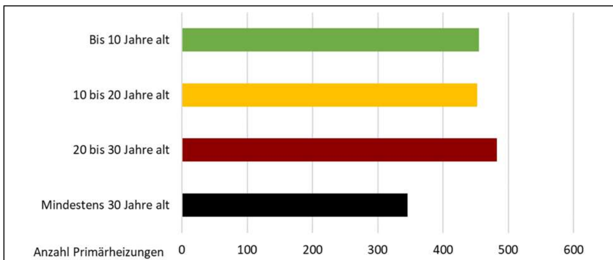
Abbildung 5 – Einbaujahr der Heizanlagen in Ehrenkirchen
